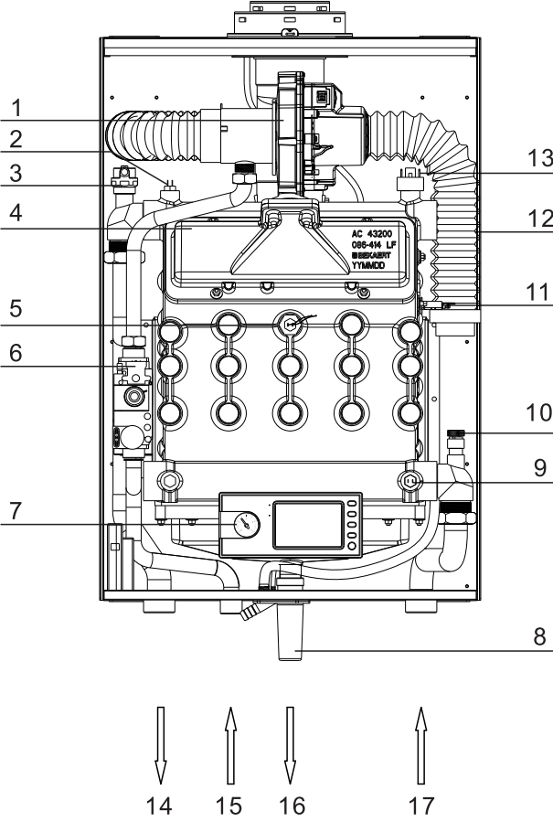
SN系列冷凝机结构示意图
