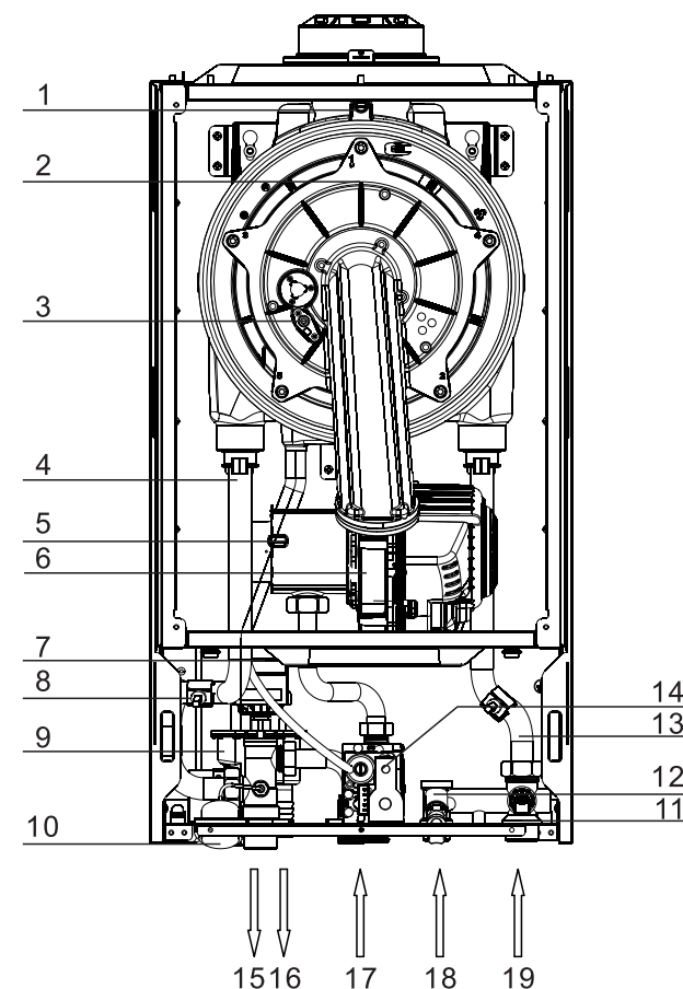
S系列冷凝机结构示意图
