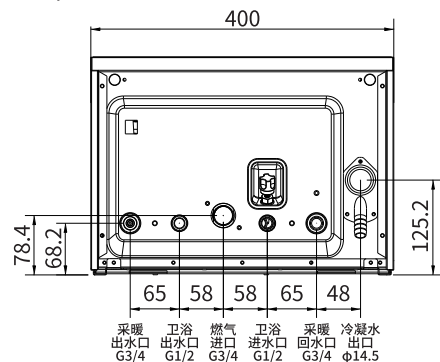
W/Me系列 冷凝机水路连接示意图
