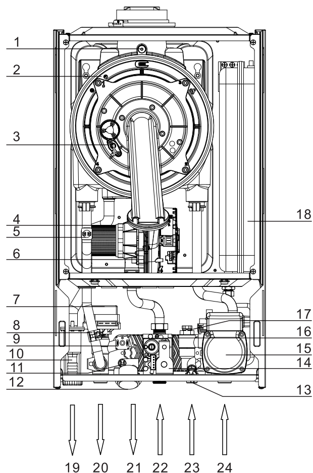
S/SP/GS系列冷凝机结构示意图
