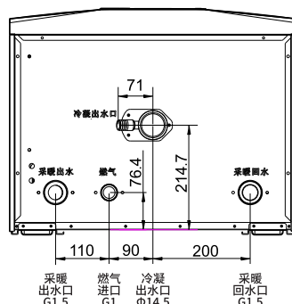
SN系列 99/120/150kW 冷凝机水路连接示意图
