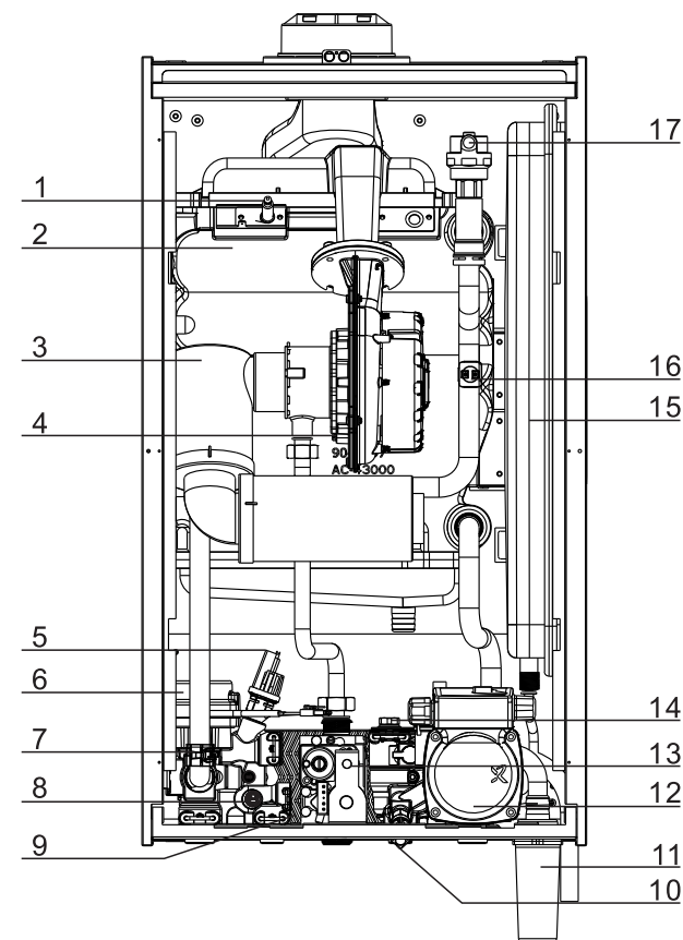
Me系列冷凝结构示意图
