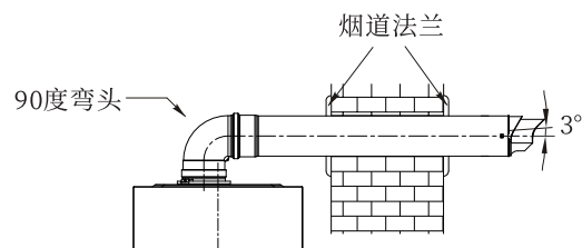
冷凝机烟道图示
