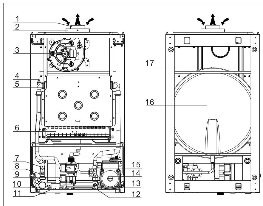
工程机型结构示意图
