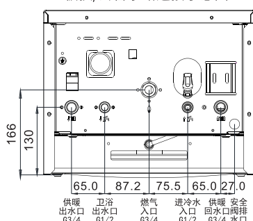
M/工程/X系列 板换/套管水路连接示意图
