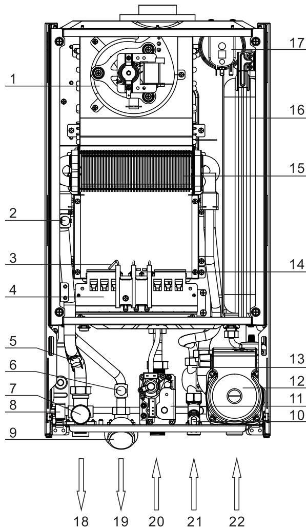
B结构小功率套管机型结构示意图
