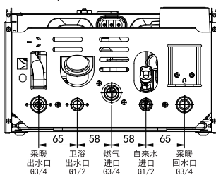
B/E/GB系列 板换/套管水路连接示意图
