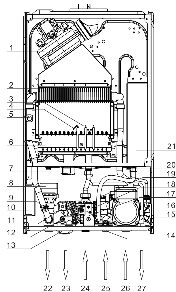
零冷水机型结构示意图
