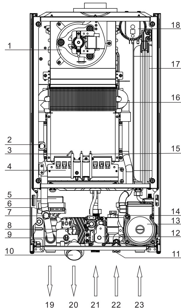
B结构小功率板换机型结构示意图
