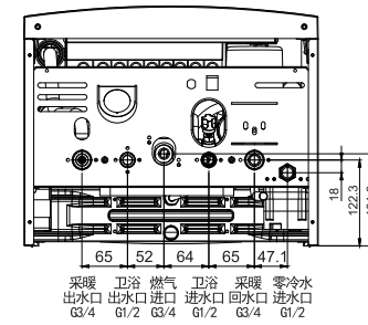
SS零冷水系列 水路连接示意图
