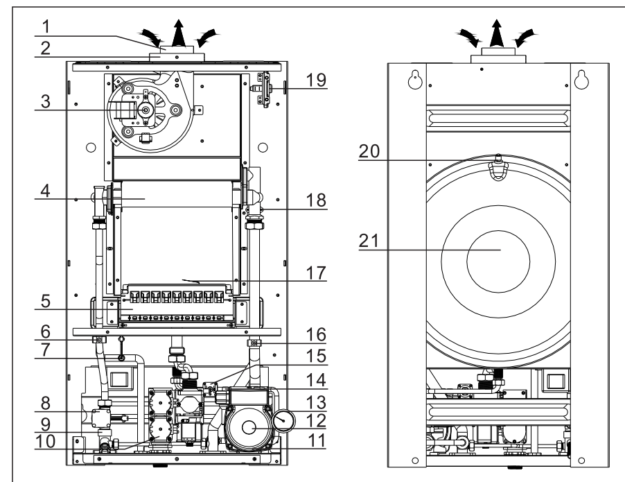
工程机型结构示意图
