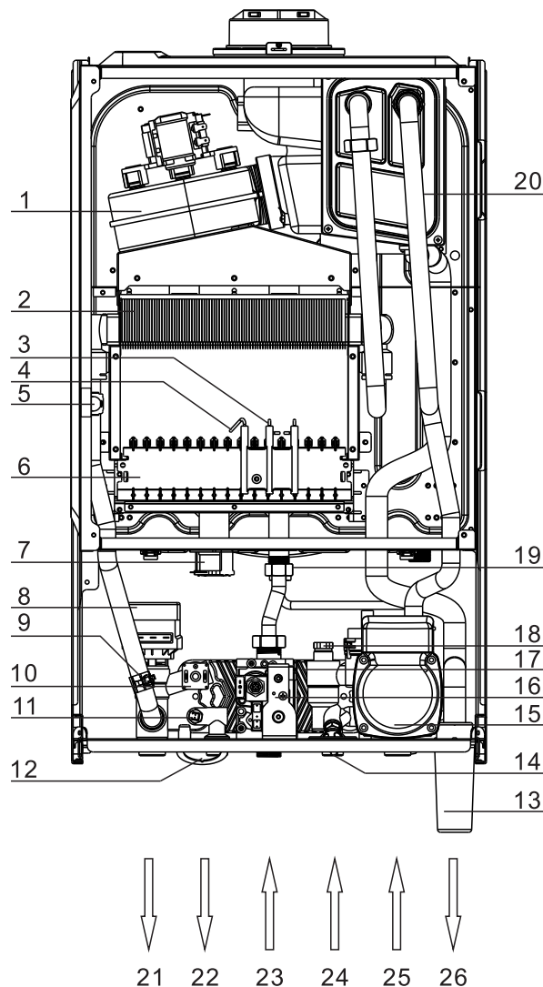
二次冷凝机型结构示意图
