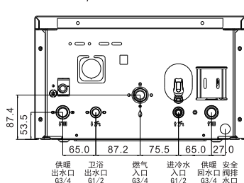
M/工程机/X系列 板换/套管水路连接示意图
