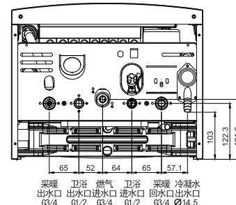
SS二次冷凝系列 水路连接示意图
