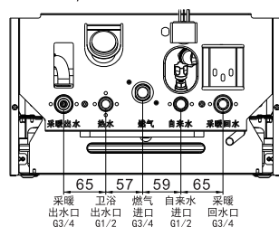
M/工程/X系列 板换/套管水路连接示意图
