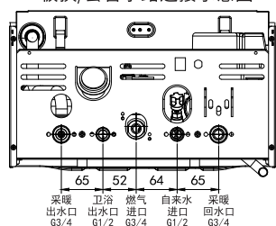
SS/C/D/S/E/C3/F/GS系列 板换/套管水路连接示意图
