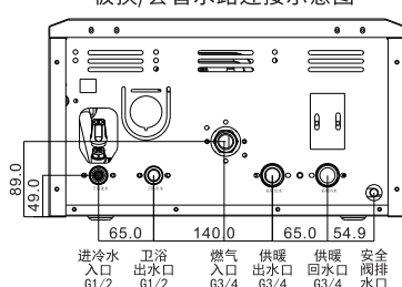
M/工程/X系列 板换/套管水路连接示意图
