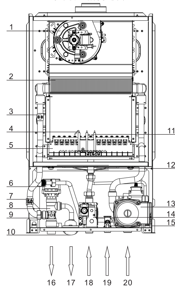
水罐机型结构示意图
