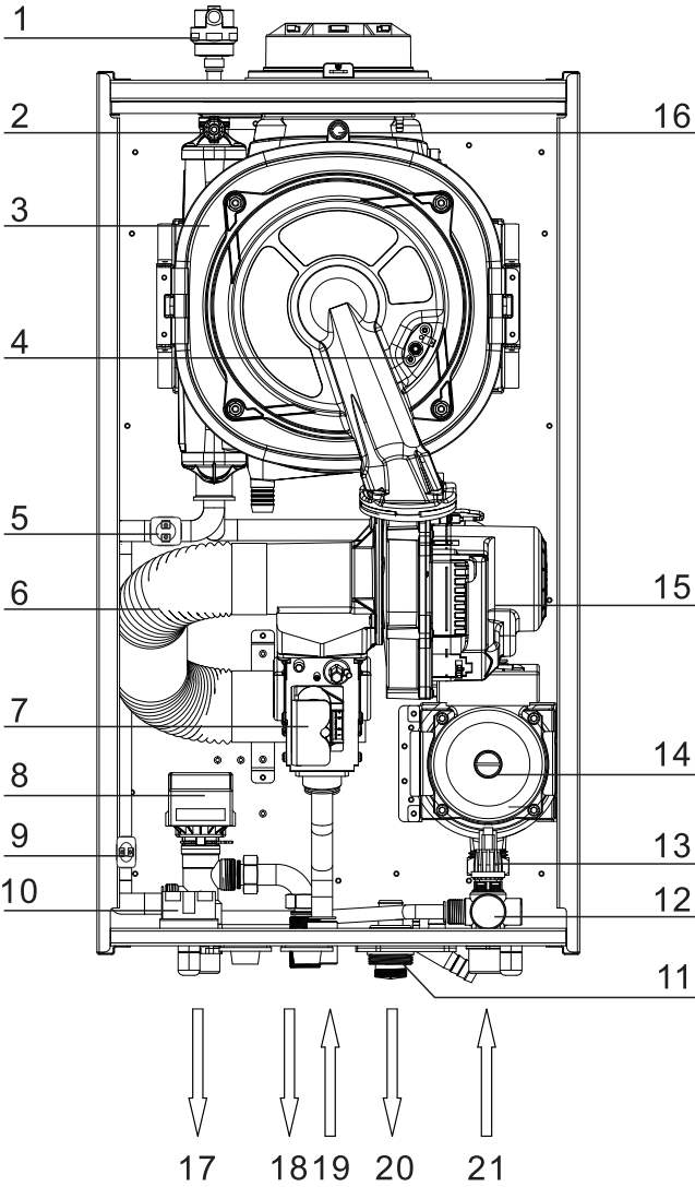
冷凝机结构示意图
