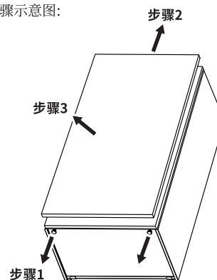
壁挂炉外壳打开 步骤示意图：
