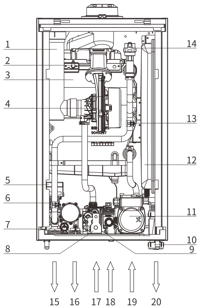
LIKE系列冷凝机结构示意图
