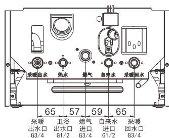
D系列水罐机 板换/套管水路连接示意图
