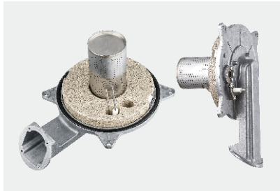
全预混燃烧技术 耐高温不锈钢
