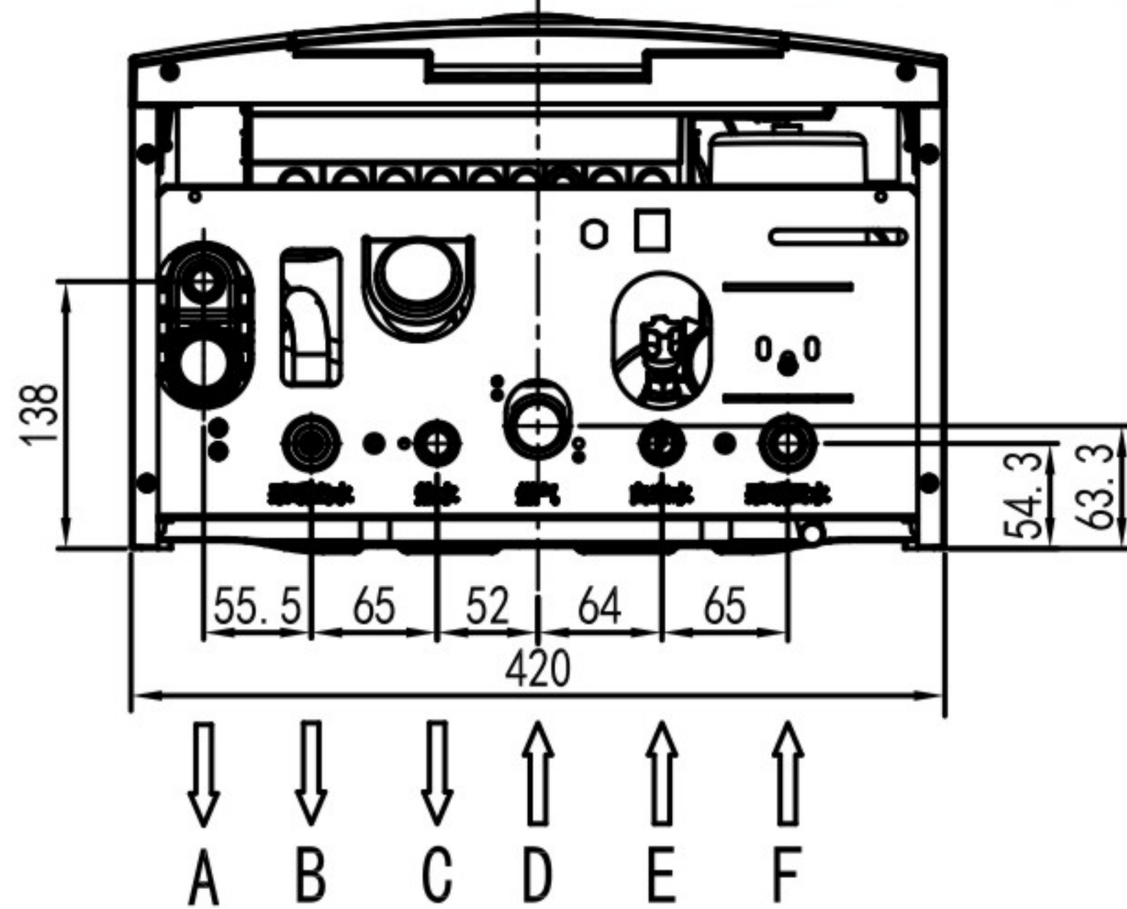
Super Plus系列 冷凝机水路连接示意图
