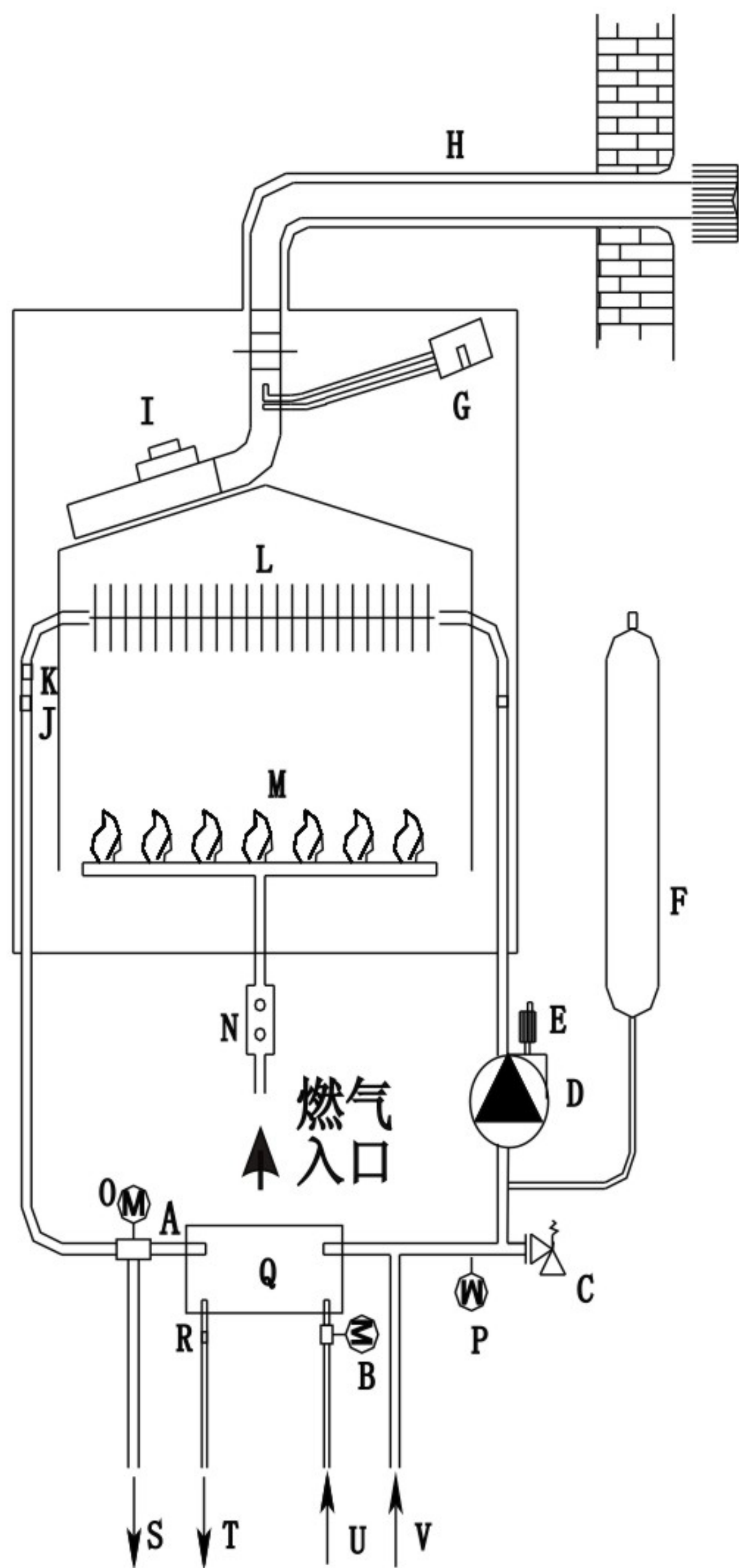
系统原理示意图
