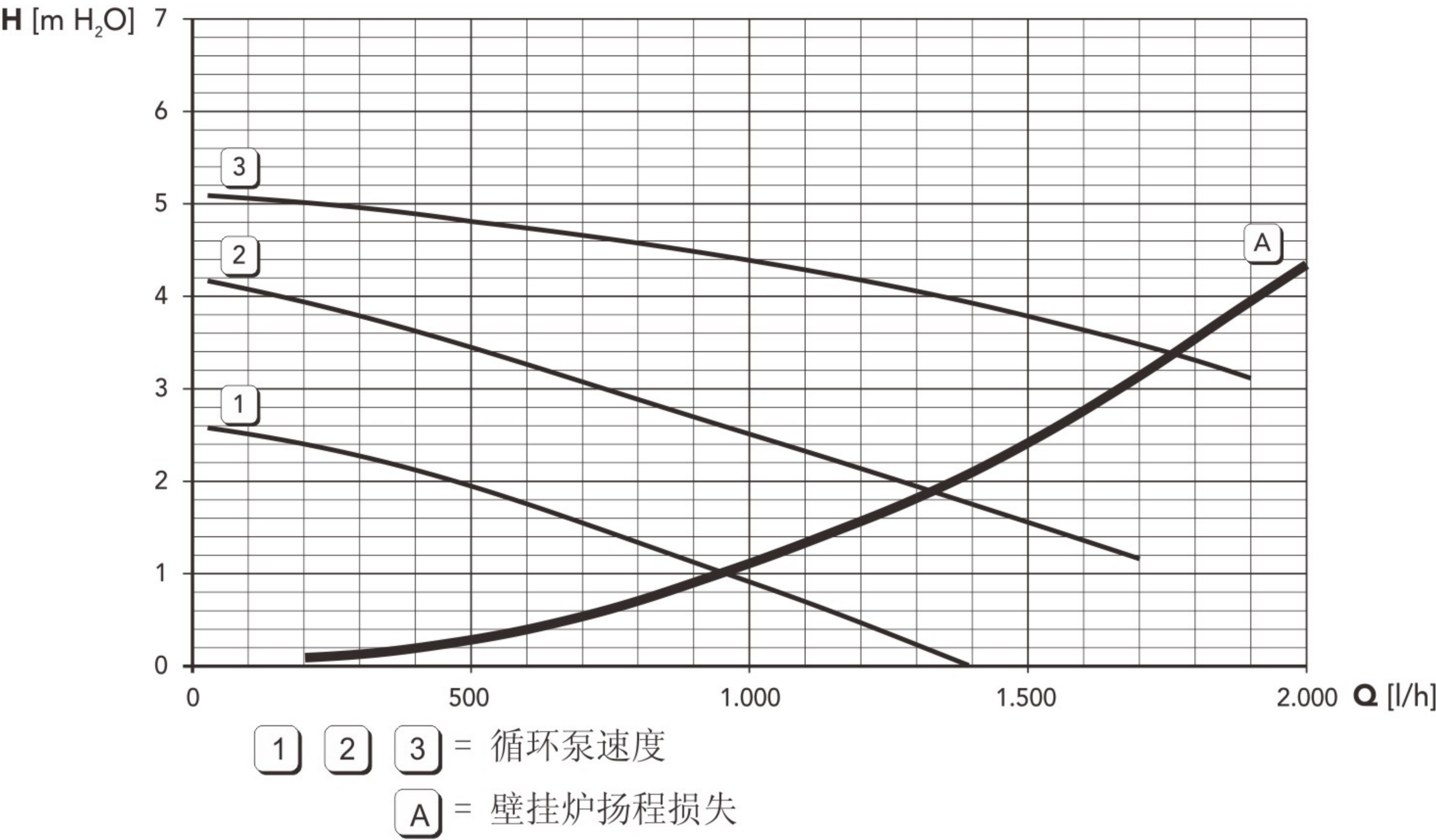
循环泵流量-扬程曲线图
