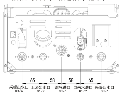
Blus/Eco系列 板换/套管水路连接示意图
