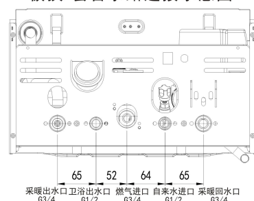
Super/Com系列 板换/套管水路连接示意图
