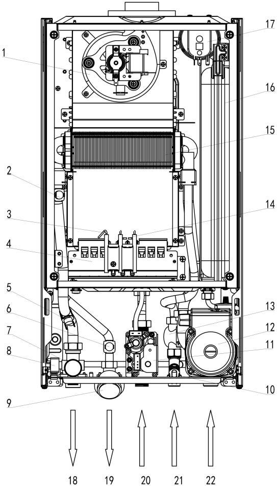
套管机型结构示意图
